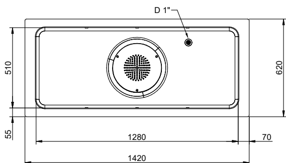
Planta
